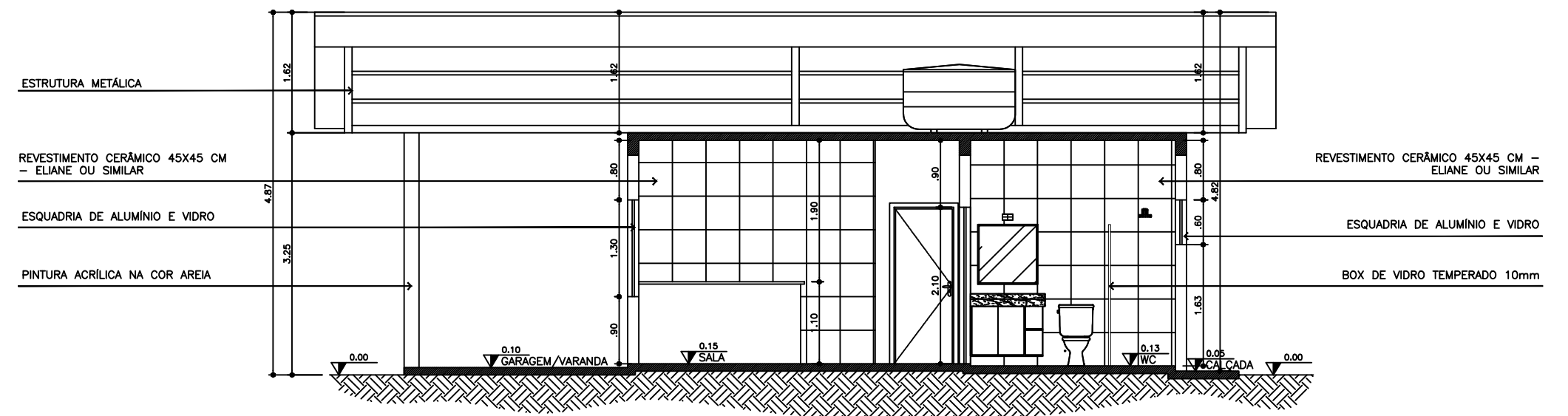
CORTE escala 1: 50
