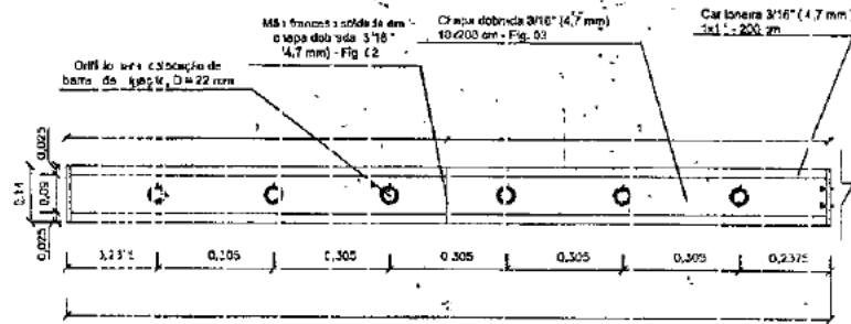
VISTA FRONTAL TRILHO DE FECHAMENTO 1 S/ESCALA
