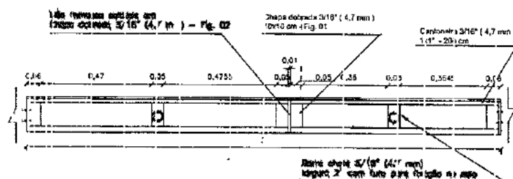
VISTA SUPERIOR TRILHO DE FECHAMENTO 2 S/ESCALA
