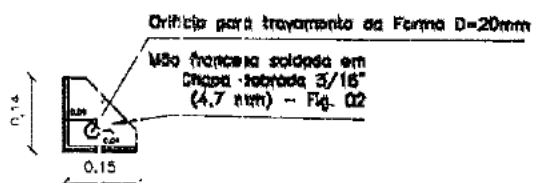
VISTA LATERAL S/ESCALA
