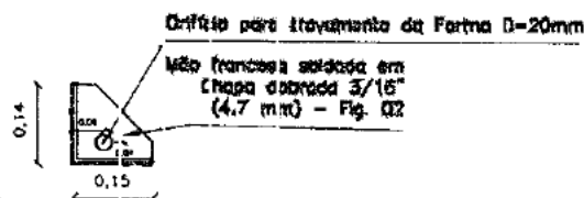
VISTA LATERAL S/ESCALA
