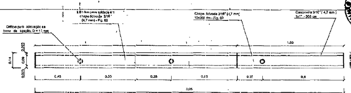
VISTA FRONTAL FORMA - TIPO 7 S/ESCALA
