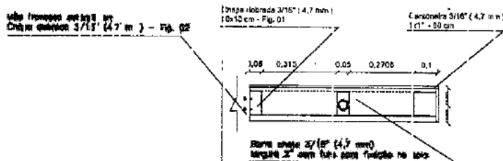
VISTA SUPERIOR TRILHO DE FECHAMENTO 3 S/ESCALA
