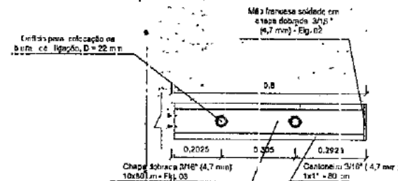
VISTA FRONTAL TRILHO DE FECHAMENTO 3 S/ESCALA
