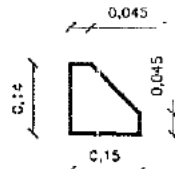
FIG. 02 - MÃO FRANCESA CHAPA 3/16" S/ESCALA
