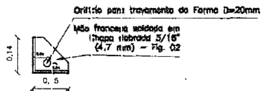
VISTA LATERAL S/ESCALA
