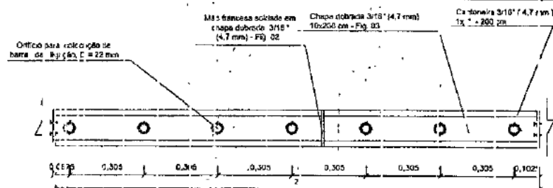
VISTA FRONTAL TRILHO DE FECHAMENTO 2 S/ESCALA
