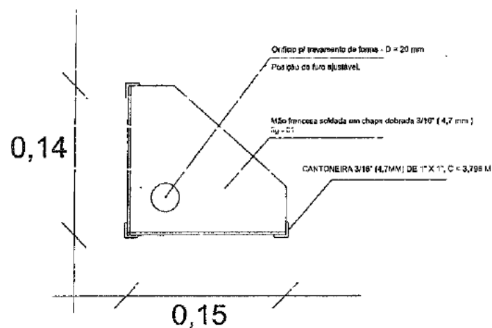
*VISTA LATERAL *S/ ESCALA
