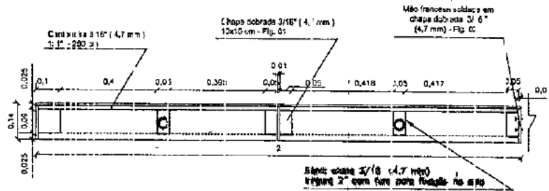
VISTA SUPERIOR TRILHO DE FECHAMENTO 1 S/ESCALA
