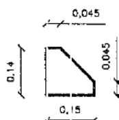
Fig. 02 - MÃO FRANCESA CHAPA 3/16" S/ESCALA
