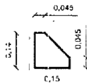
FIG. 02 - MÃO FRANCESA CHAPA 3/16" S/ESCALA
