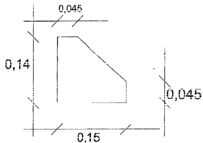
*FIGURA 01 - Mão francesa chapa \frac{3}{16} " (4,7 mm) *S/ ESCALA
