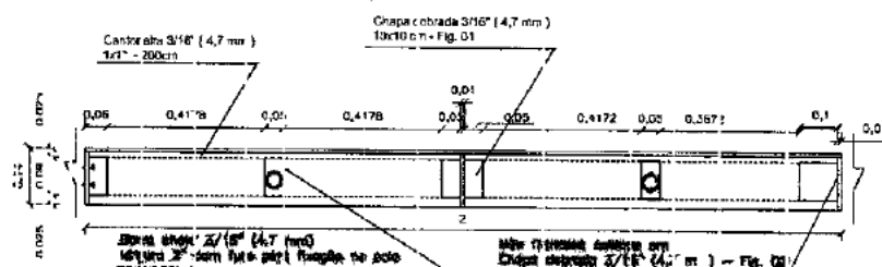
VISTA SUPERIOR TRILHO DE FECHAMENTO 5 S/ESCALA
