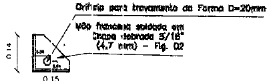
VISTA LATERAL S/ESCALA
