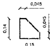
FIG. 02 - MÃO FRANCESA EM CHAPA 3/16\"/>
