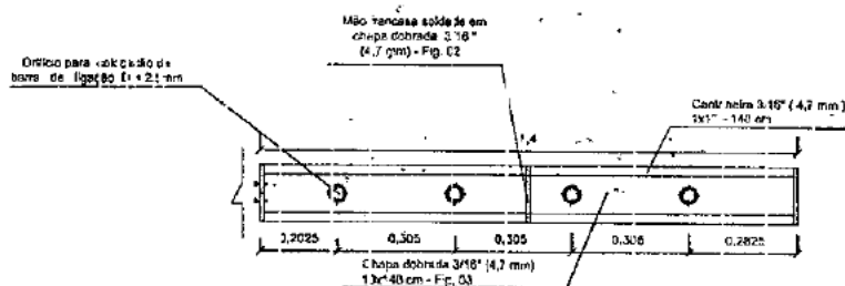
VISTA FRONTAL TRILHO DE FECHAMENTO 4 S/ESCALA
