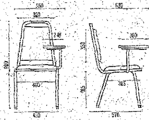
1001 U Empilhável com Prancheta
