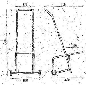
1100 Carrinho para Transporte
