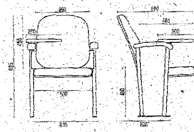
12011 UE Auditório com Prancheta
