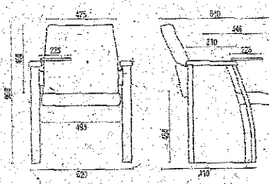
12020 UE Auditório com Prancheta
