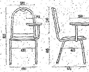
1002 U Empilhável com Prancheta
