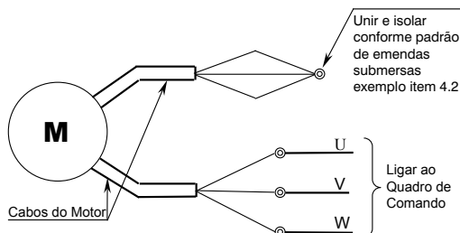
Figura 6.5.4 - Motor com dupla Tensão - Ligação 380V
