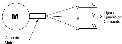
Figura 6.5.1 - Motor com um cabo chato ou 3 unipolares
