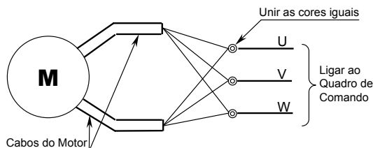
Figura 6.5.3 - Motor com dupla Tensão - Ligação 220V
