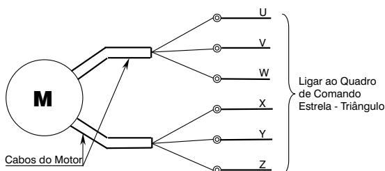
Figura 6.5.5 - Ligação de Motores para Partida Estrela - Triângulo
