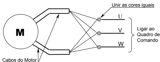
Figura 6.5.2 - Motor com dois cabos (Tensão Fixa)
