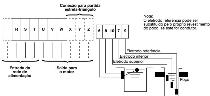
Figura 6.6 - Conexão do Quadro de Comando
