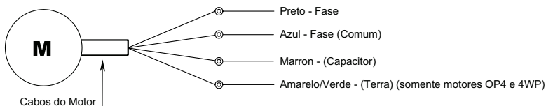
Figura 6.5.6 - Ligação de Motores Monofásicos
