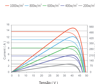
Curvas de corrente-tensão e potência-tensão (540W)
