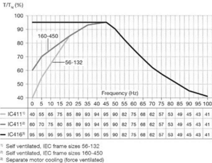
Figura 6a. Outros conversores de alimentação tipo PWM, 50 Hz, aumento de temperatura B
