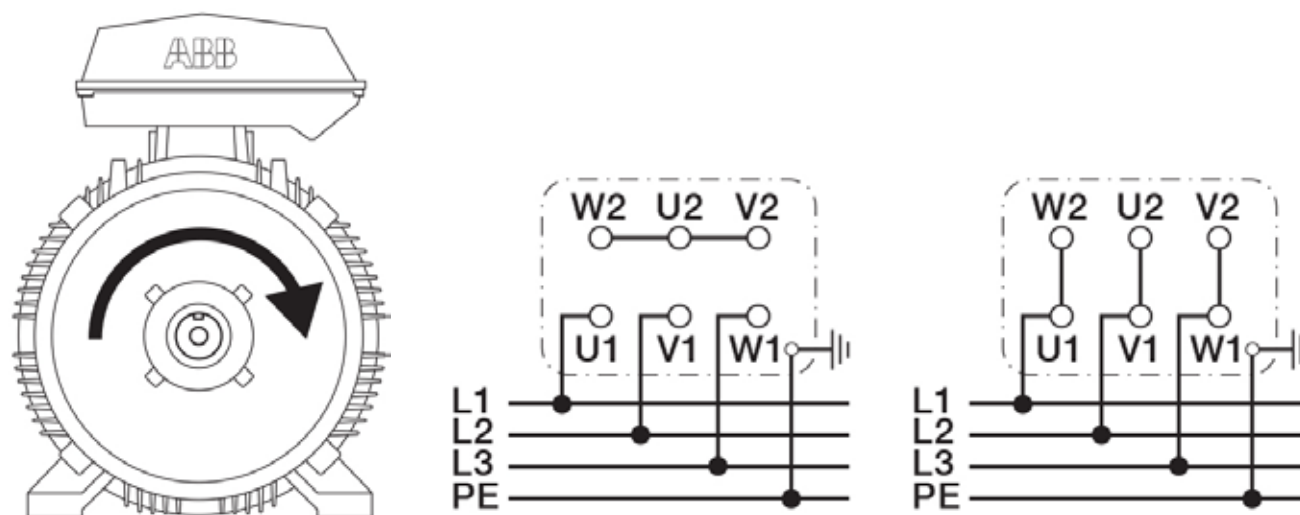
Figura 3. Ligação de terminais para alimentação
