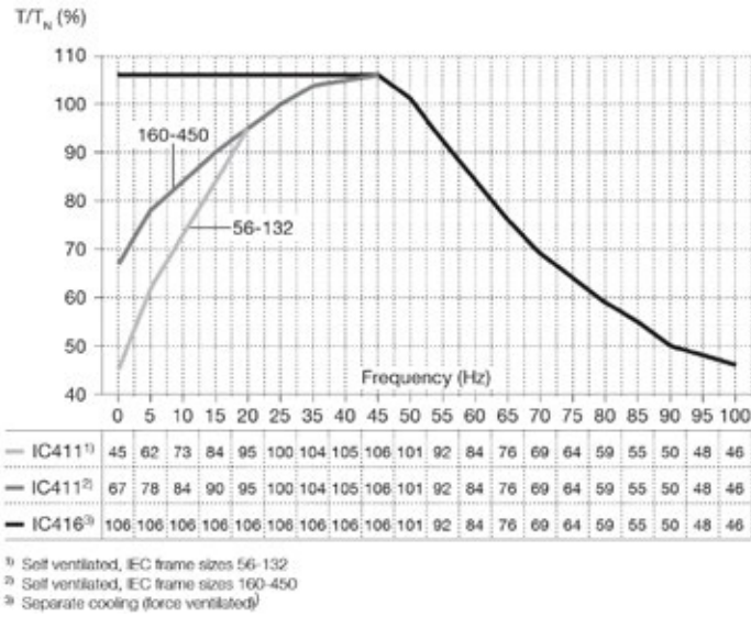
Figura 6c. Outros conversores de alimentação tipo PWM, 50 Hz, aumento de temperatura F
