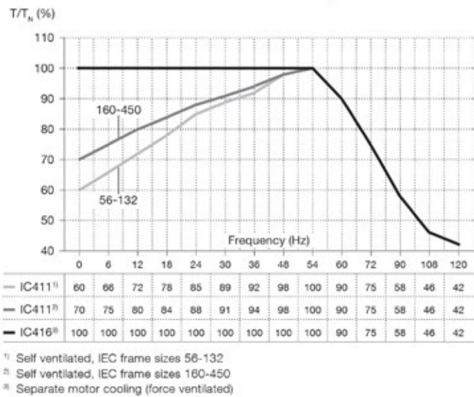
Figura 5b. Conversor com controlo DTC, 60 Hz, aumento de temperatura B
