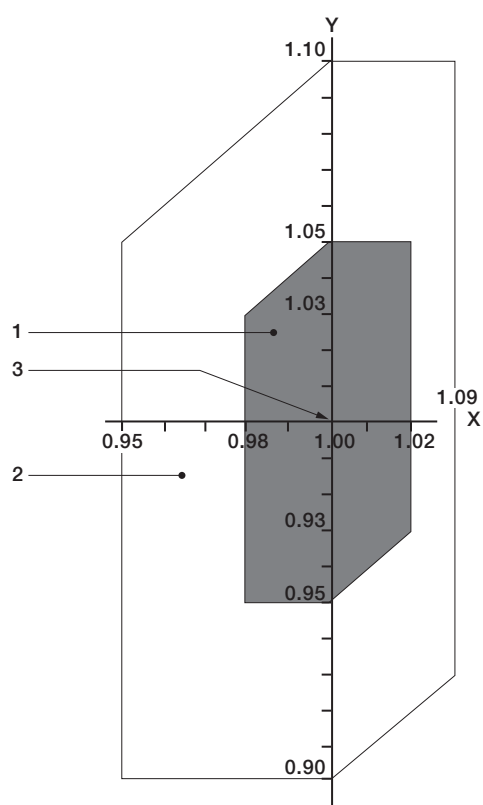
Figura 4. Desvio de tensão e frequência nas zonas A e B
