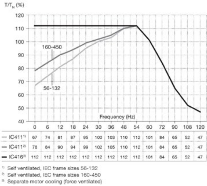
Figura 5d. Conversor com controlo DTC, 60 Hz, aumento de temperatura F
