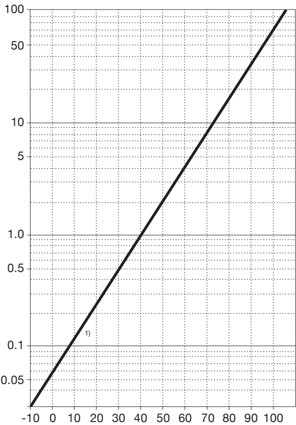
Figura 1. Diagrama que ilustra a dependência da resistência de isolamento em relação à temperatura, e como corrigir a resistência de isolamento medida para a temperatura de 40 °C.
