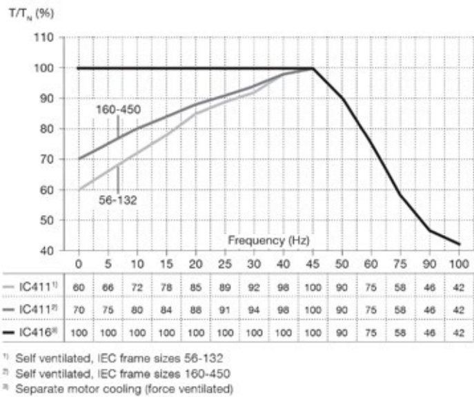
Figura 5a. Conversor com controlo DTC, 50 Hz, aumento de temperatura B
