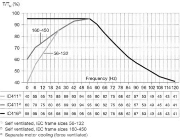
Figura 6b. Outros conversores de alimentação tipo PWM, 60 Hz, aumento de temperatura B
