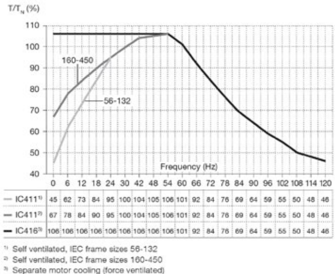
Figura 6d. Outros conversores de alimentação tipo PWM, 60 Hz, aumento de temperatura F
