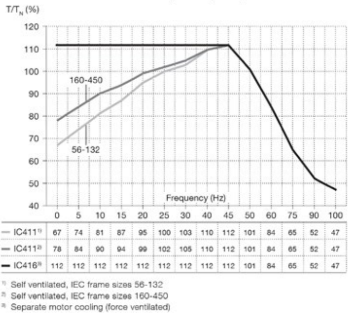
Figura 5c. Conversor com controlo DTC, 50 Hz, aumento de temperatura F
