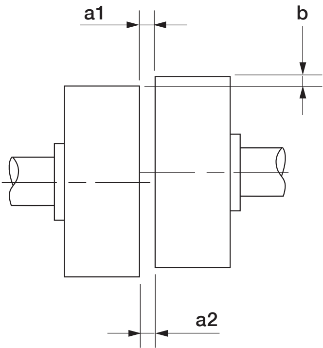
Figura 2. Montagem dos meios-acoplamentos ou polias
