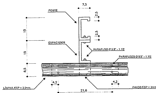
ESQUEMA DE FIXAÇÃO POSTE/ESPAÇADOR/LÂMINA
