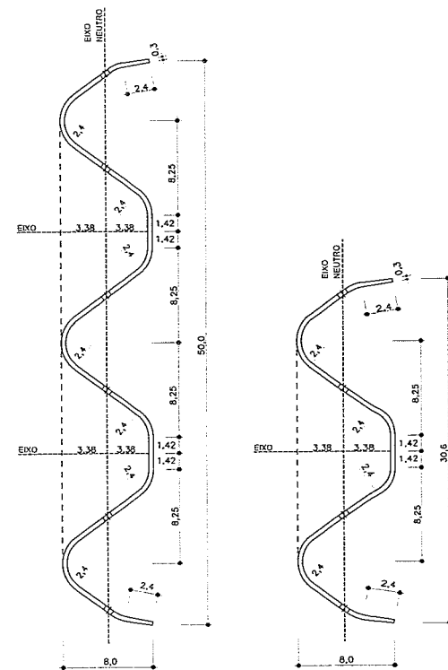
LÂMINA TRIPLA ONDA
