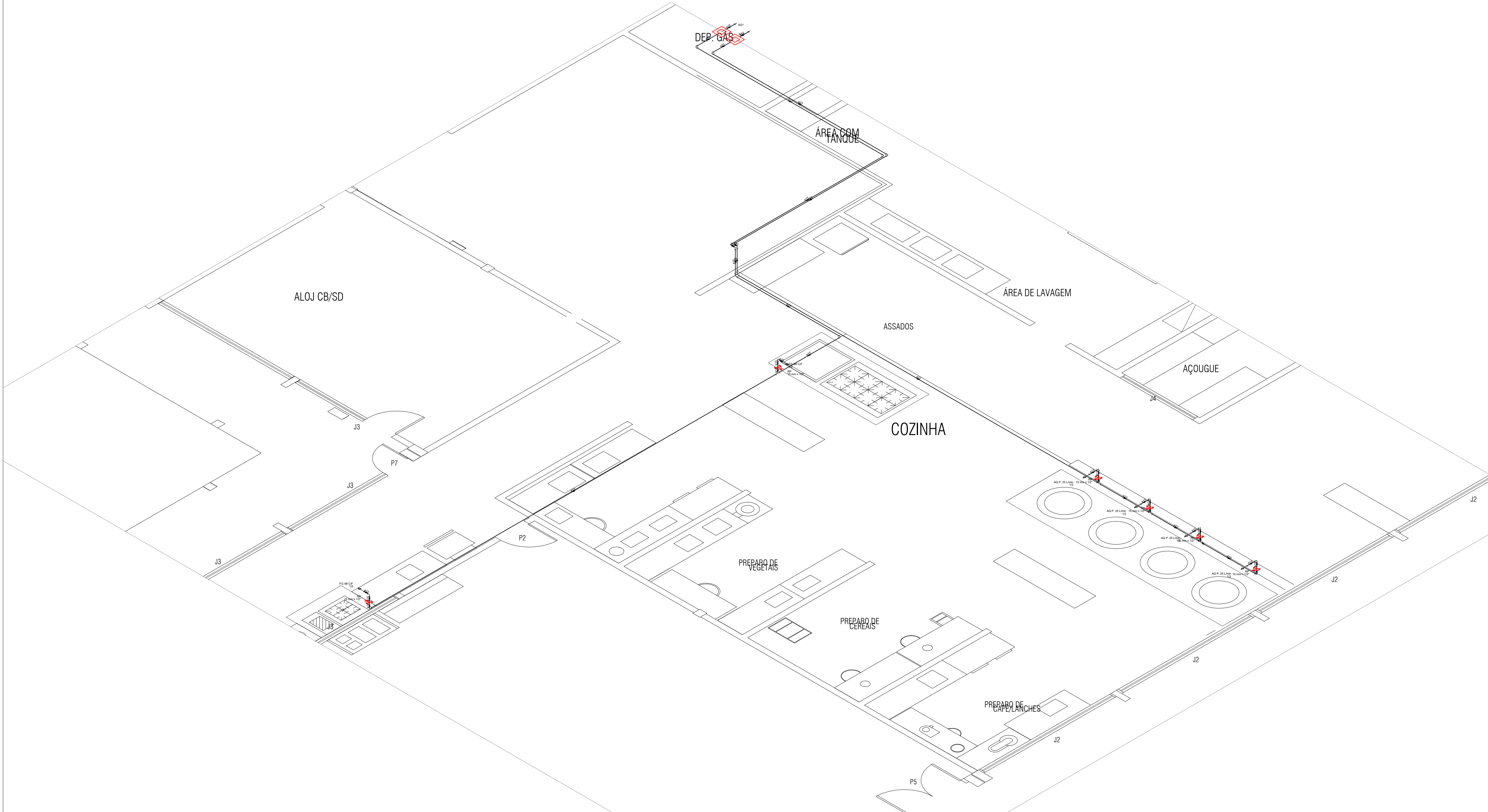
2 02 - ISOMÉTRICO GÁS-1 escala 1 : 150
