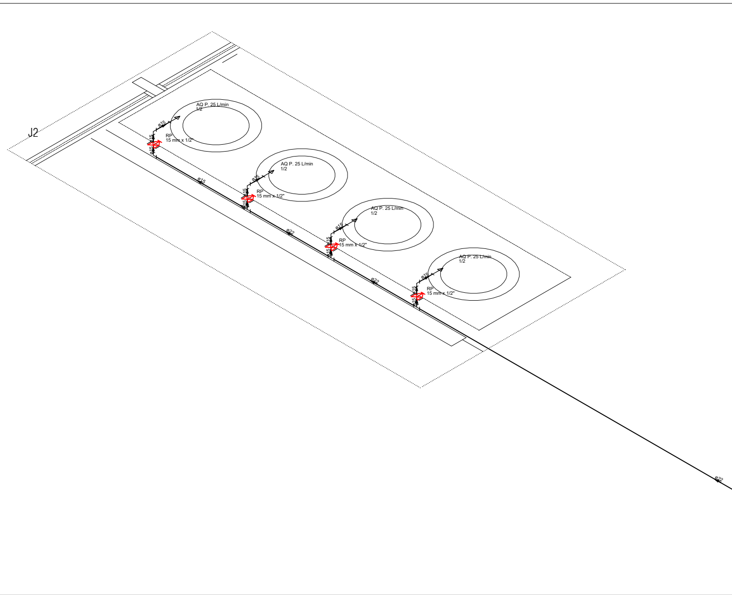
3 03 - ISOMÉTRICO GÁS escala 1 : 150
