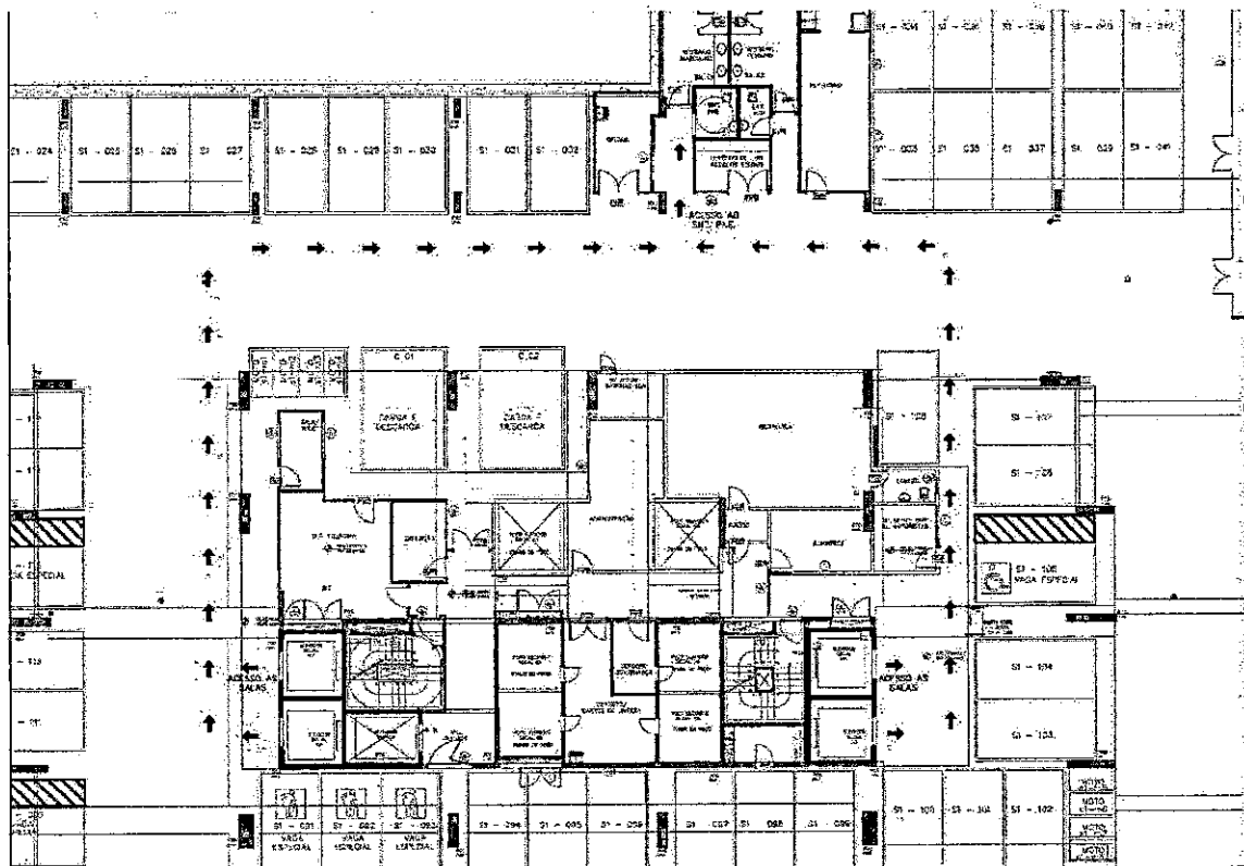
Figura 1 - Planta esquemática 1º subsolo
