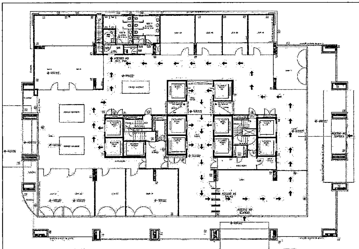
Figura 2 - Planta esquemática térreo
